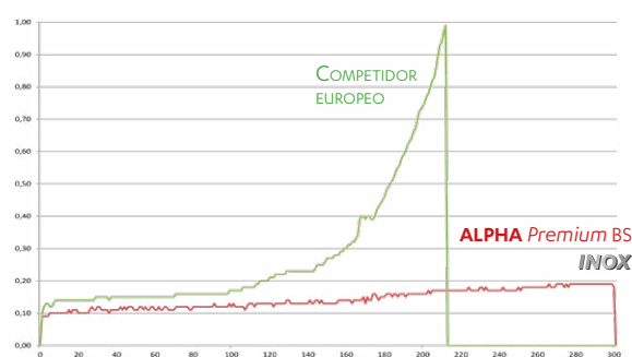
Prueba comparativa de desgaste de una cadena Alpha Premium INOX con una cadena Inox alta gama europea
