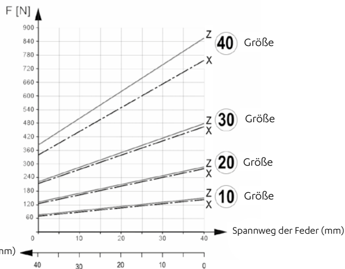
Belastungsdiagramm
