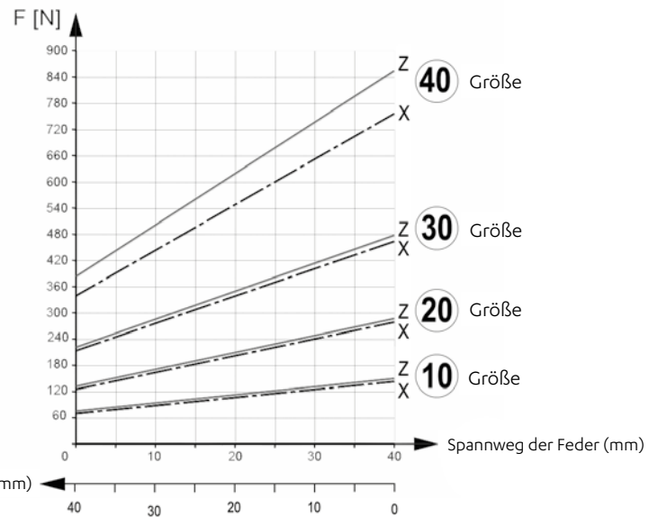
Belastungsdiagramm
