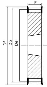
Typ 4F Vollscheibe mit Bordscheiben
