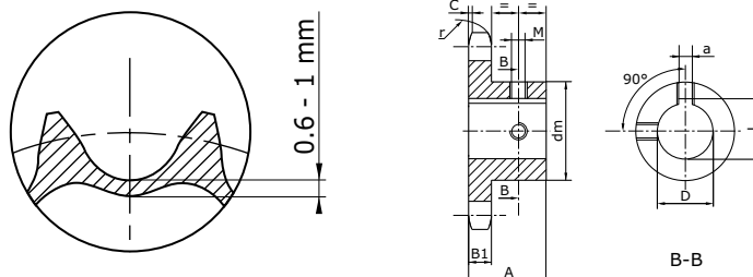
Für Abmessungen a, L und M siehe Tabelle Seite 103
