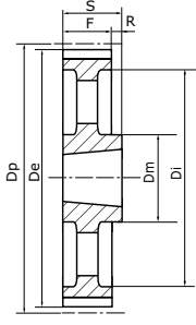
Typ 8E Hohl-Riemenscheibe
