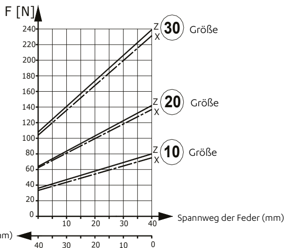
Belastungsdiagramm
