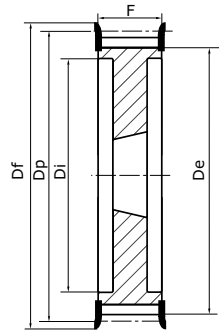
Typ 5F Vollscheibe mit Bordscheiben
