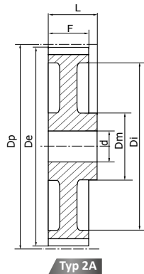
Typ 2A leichtere Riemenscheibe
