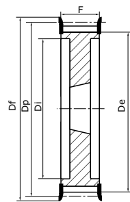
Typ 5F Vollscheibe mit Bordscheiben
