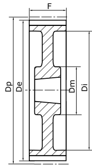
Typ 9A leichtere Riemenscheibe
