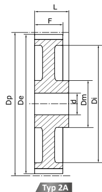
Typ 2A leichtere Riemen-scheibe
