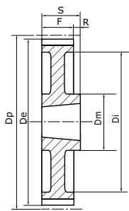
Typ 8A leichtere Riemenscheibe
