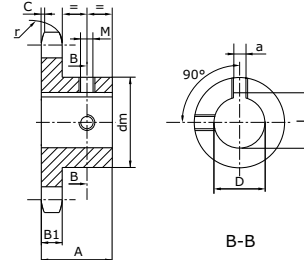
Für Abmessungen a, L und M siehe Tabelle Seite 103
