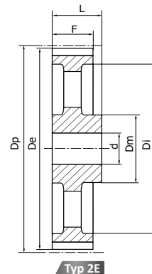
Typ 2E Hohl-Riemen-scheibe
