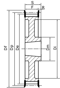
Typ 8AF leichtere Riemenscheibe
