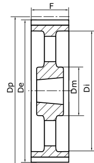
Typ 9E Hohl-Riemenscheibe
