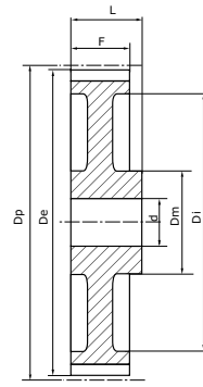
Type 2A leichtere Riemenscheibe
