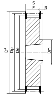
Typ 8F Vollscheibe mit Bordscheiben
