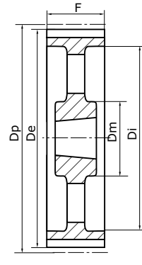
Typ 9E Hohl-Riemenschleibe
