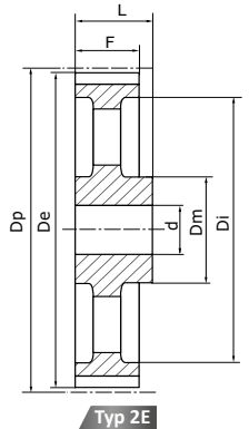
Typ 2E Hohl-Riemenscheibe
