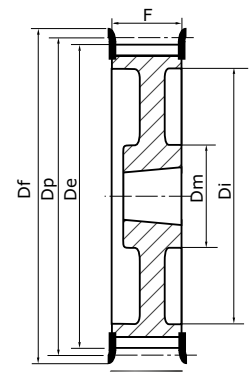
Typ 6AF leichtere Riemenscheibe
