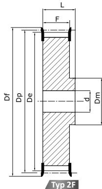
Typ 2F Vollscheibe mit Bordscheiben
