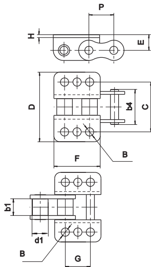
Cadenas 2060 con aletas K5
