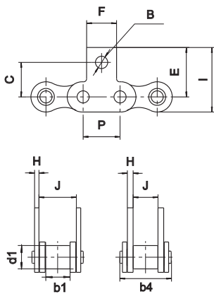
M1C: Aleta corta con 1 taladro
