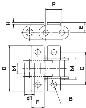
K1C: Aleta corta con 1 taladro
