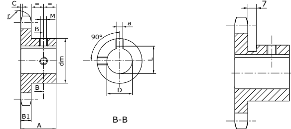
Pour les côtes a, L et M voir tableau page 103
