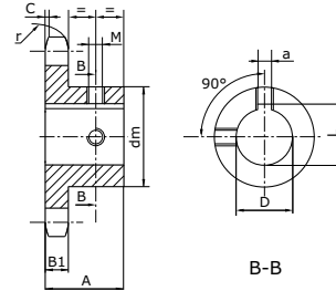
Pour les côtes a, L et M voir tableau page 103
