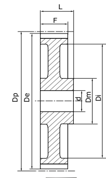
Type 2A Poulie allégée non flasquée
