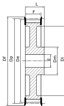
Type 2AF Poulie allégée flasquée
