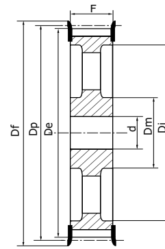
Type 3EF Poulie évidée flasquée
