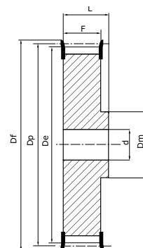
Type 2F Poulie pleine flasquée
