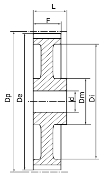
Type 2A Poulie allégée non flasquée
