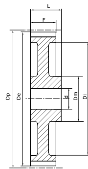
Type 2A Poulie allégée non flasquée
