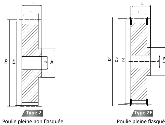
Type 2 Poulie pleine non flasquée
